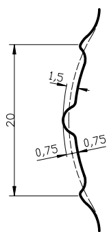
SECCION.-A-A
