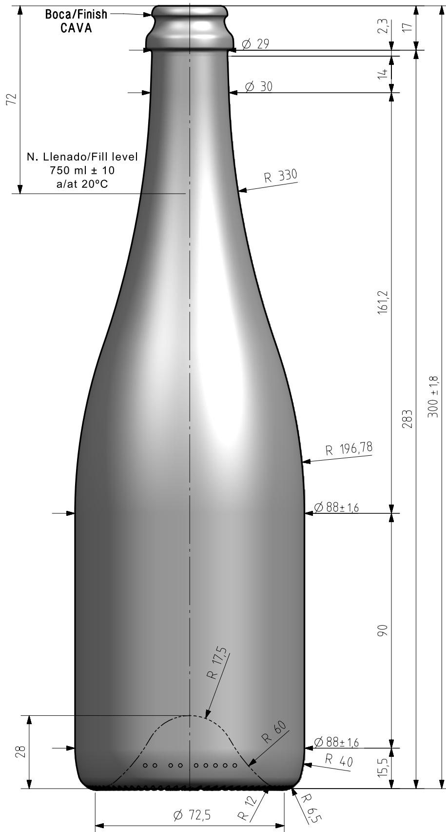
ZONA DE GRABADOS / HEEL EMBOSING (Opuesto al código de pts / Opposite to dot code)
