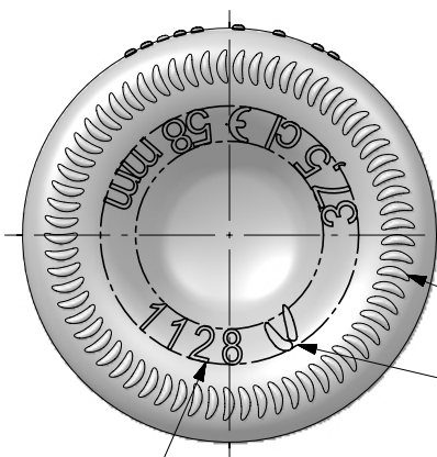
N.º MODELO (JOB No) VISTA DEL FONDO (BOTTOM VIEW)
